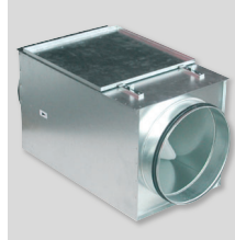
MFL-F Caisson filtre pour filtres à poches F5, F6 ou F7.
