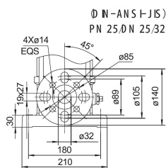
Bride DIN (/F)
