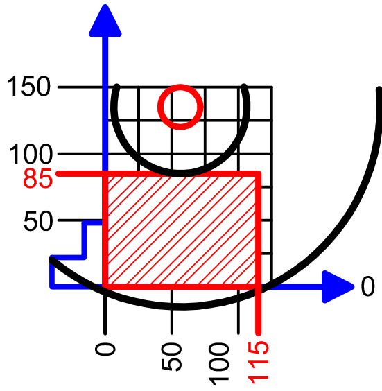
90° : 115 x 85 mm.
